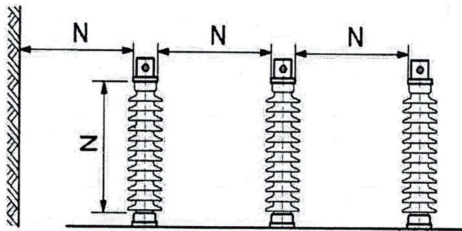
Hình 3.1: Khoảng trống cách điện nhỏ nhất (N) giữa các phần mang điện và giữa các phần mang điện với đất đối với thanh cái cứng
