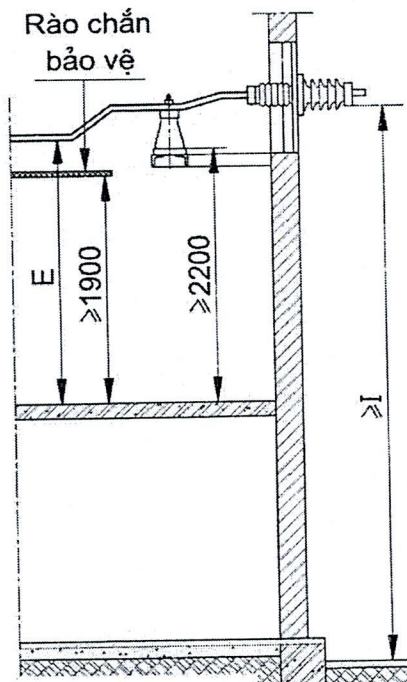
Hình 3.10: Chiều cao nhỏ nhất trên hành lang đi lại trong nhà và khu vực không có đường đi lại bên ngoài TBA
