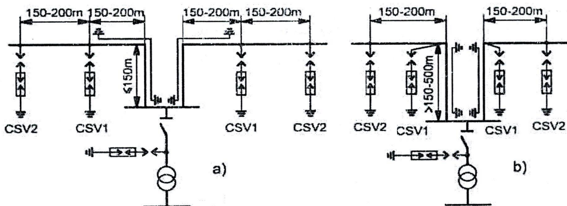
a) Nhánh rẽ dài đến 150m b) Nhánh rẽ dài trên 150m đến 500m
